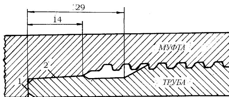
1 – торцеве упорне ущільнення; 2 – бокове кінцеве ущільнення
