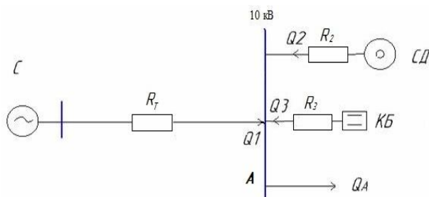
Рисунок 2 – Розрахункова схема
