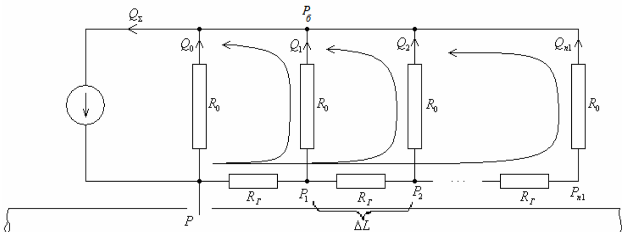
Рисунок 2 – Структурна схема моделі витоку газу вздовж газопроводу
