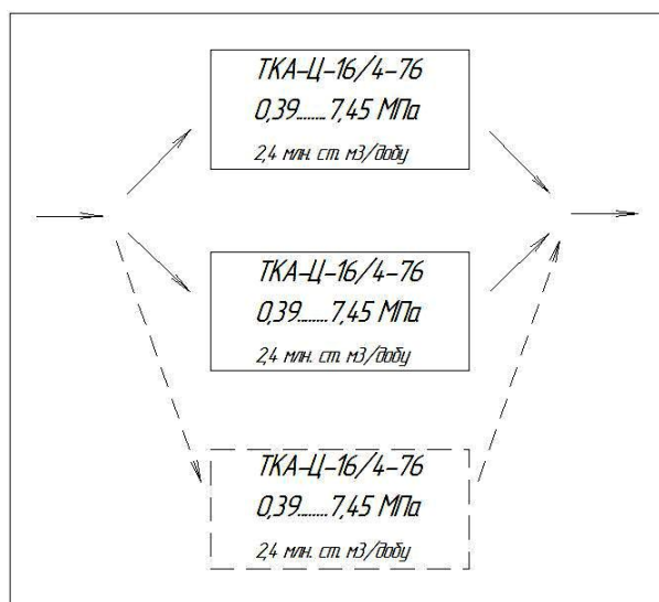
Рисунок 2 – Компонувальна схема компресорної станції для реалізації процесу розвантаження газу річною продуктивністю 2 млрд.м 3 (варіант компоновки Т1-Р)
