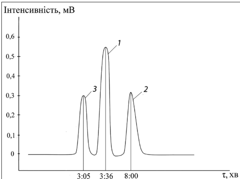
Рис. 3. Хроматограма продуктів електровідновлення ізовалеріанового альдегіду на алюмінієвому катоді із постійним контрольованим потенціалом ( E=-0,75 В): 1 – ізопропіловий спирт (розчинник); 2 – ізовалеріановий альдегід; 3 – ізопентан
