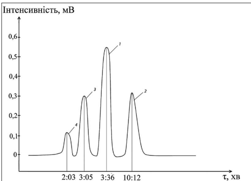
Рис. 4. Хроматограма продуктів електровідновлення петанону-2 у сірчаноокислому водно-спиртовому розчині із постійним контрольованим потенціалом ( E=-0,6 В): 1 – ізопропіловий спирт (розчинник); 2 – петанон-2, 3 – петан; 4 – пентен
