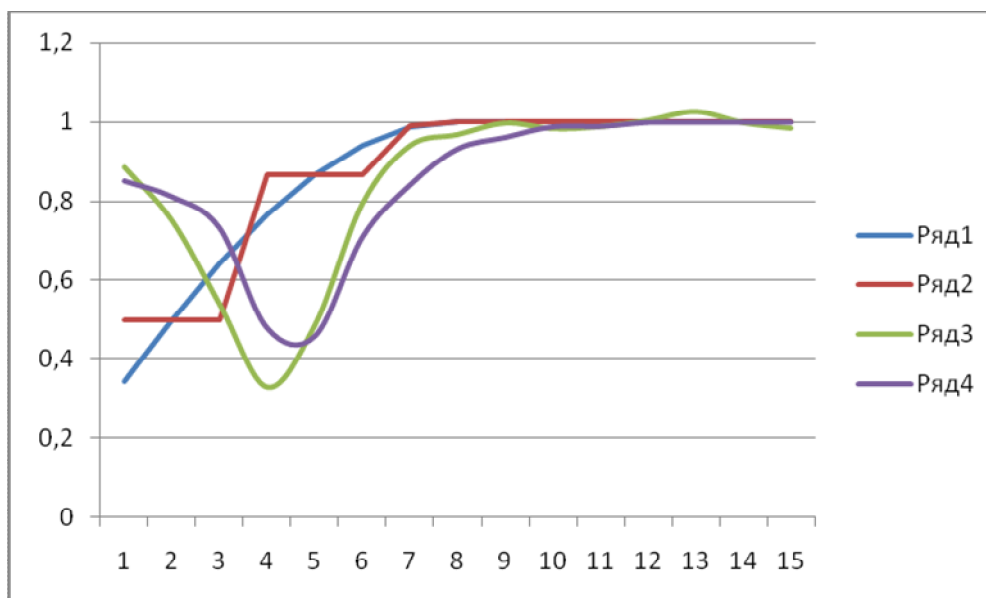
1 – крива газоспоживання; 2 – кусково-постійна апроксимація кривої газоспоживання; 3 – відносна витрата газу на початку ділянки при заданій функції газоспоживання; 4 – відносна витрата газу на початку ділянки при кусково-постійній апроксимації
