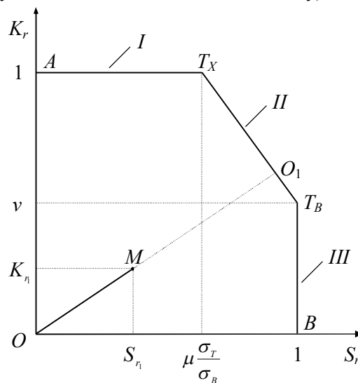
Рисунок 2 – Схематична діаграма оцінки руйнування [38]
