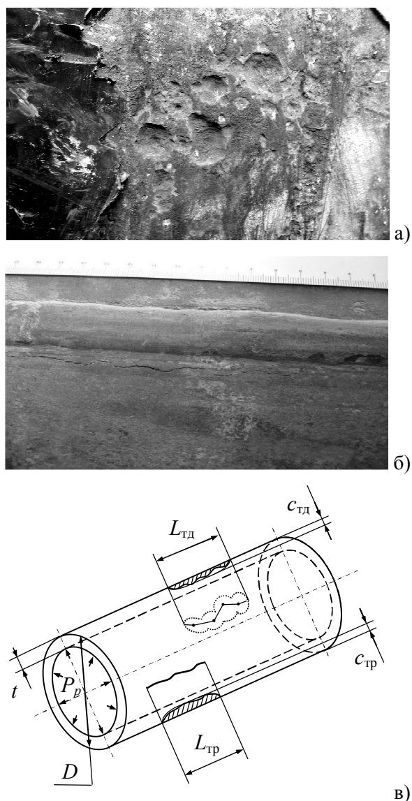
Рисунок 1 – Зовнішні експлуатаційні корозійно-механічні тріщиноподібні дефекти (а) та корозійно-втомні тріщини (б) і їх схематичне подання (в) у стінці газопровідної труби
