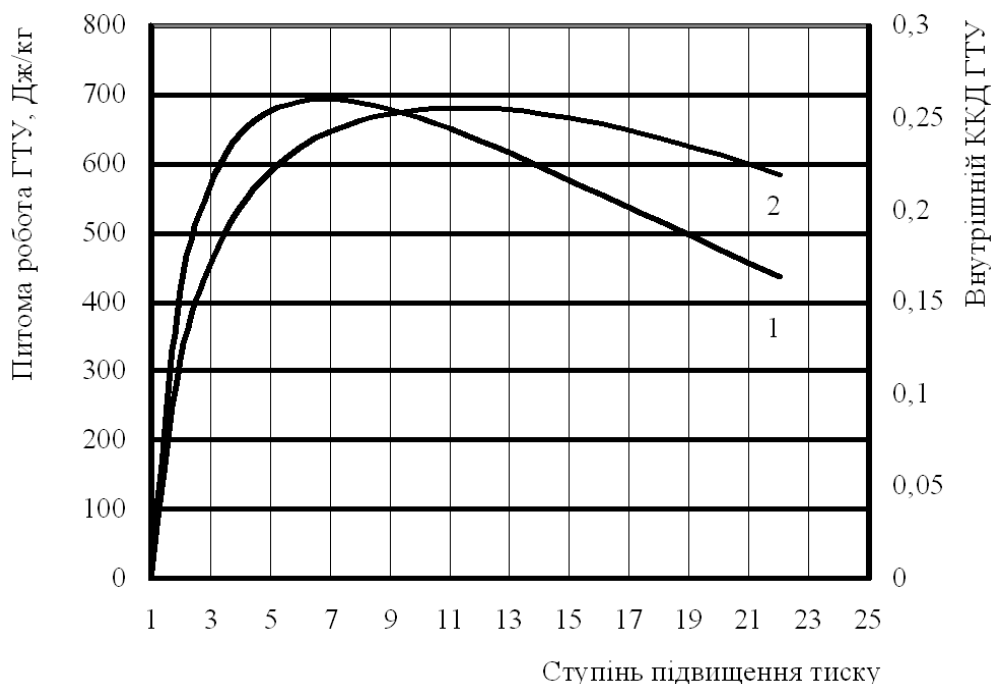
1 – питома корисна робота ГТУ; 2 – внутрішній ККД ГТУ Рисунок 1 – Залежність питомої корисної роботи ГТУ і внутрішнього ККД від ступеня підвищення тиску в осьовому компресорі
