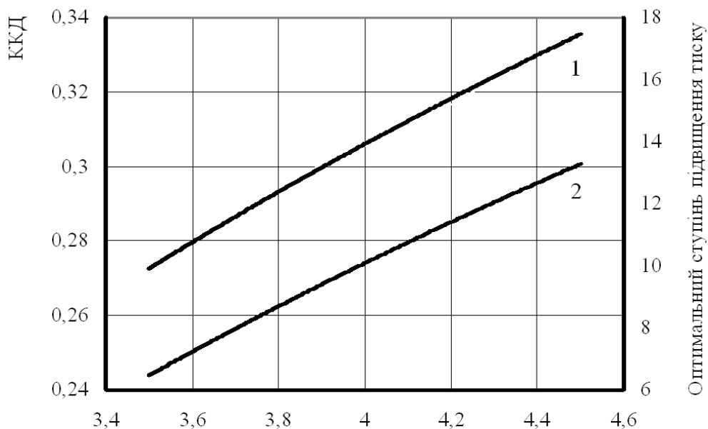
Відношення максимальної температури в циклі до мінімальної 1 – ступінь підвищення тиску; 2 – внутрішній відносний ККД ГТУ Рисунок 2 – Залежність характеристик ГТУ від відношення максимальної температури в циклі до мінімальної
