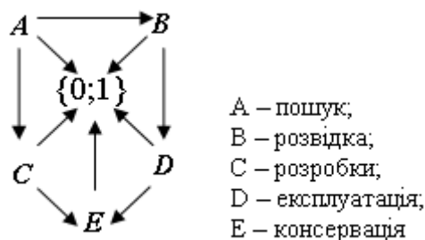
Рисунок 5 — Моделювання життєвого циклу нафтового чи газового родовища за допомогою Set-категорії
