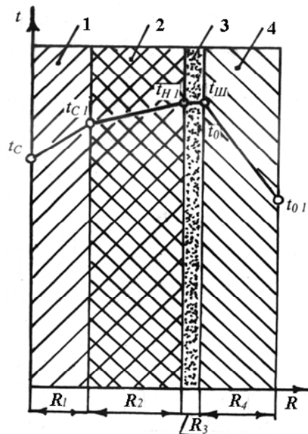
1 – основание тормозной колодки; 2,3 – фрикционная накладка и ее приповерхностный слой; 4 – обод тормозного барабана Рисунок 7 – Тепловая модель фрикционного узла барабанно-колодочного тормоза
