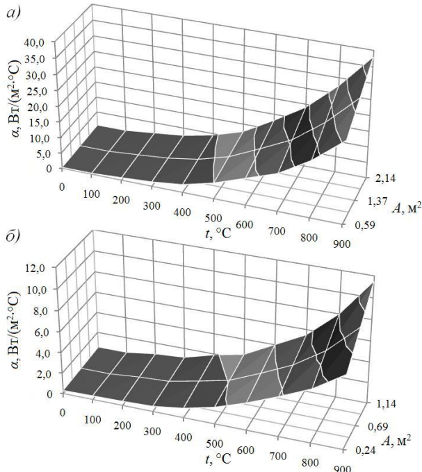
Рисунок 8 – Зависимость коэффициентов теплоотдачи (а) лучеиспусканием матовых (а) и полированных (б) поверхностей (б) от температуры нагрева (t) различных их площадей (A)
