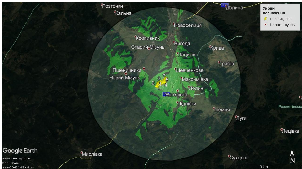
Рис. 1. Зона видимості з ВЕУ 6 ВЕС Шевченкове-1 висотою 50 м.
